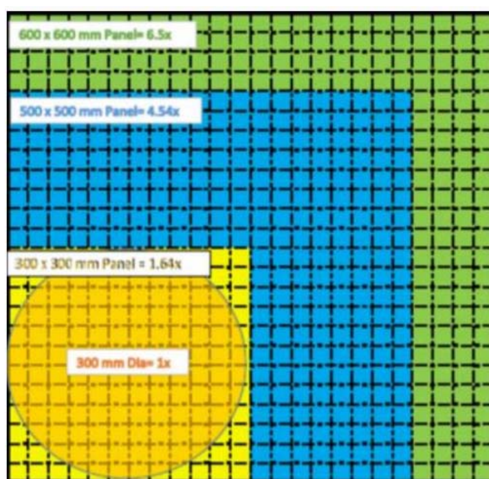
圖 10 面板級封裝示意圖
