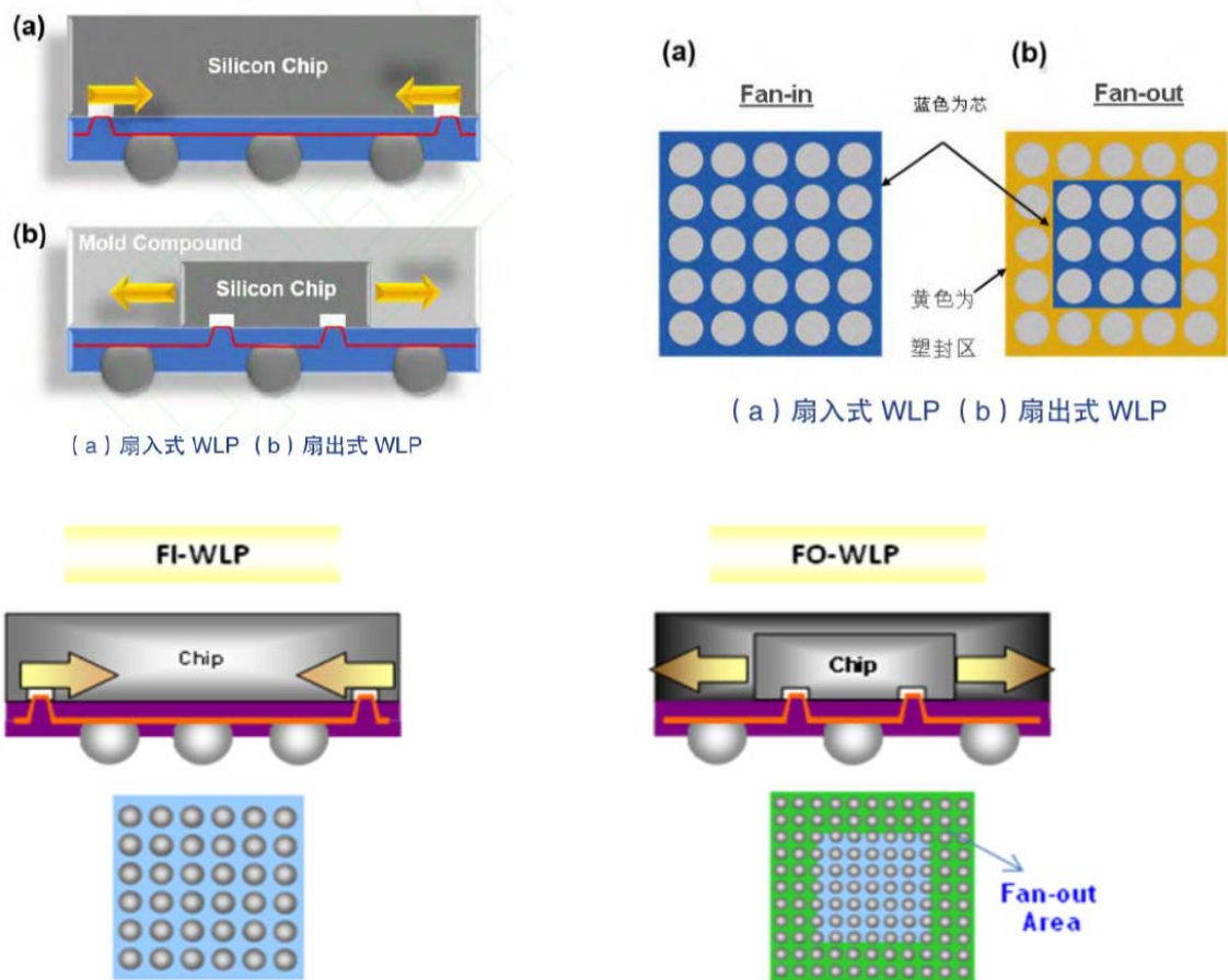
圖 8 扇入型與扇出型對比圖
