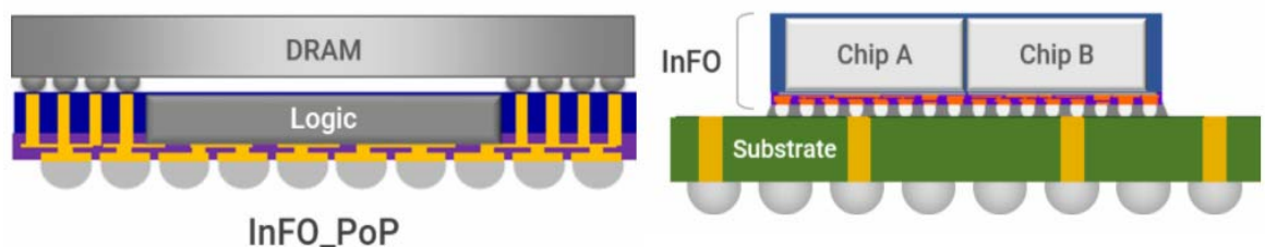
圖 9 InFO(台積電)-InFO_PoP & InFO_oS
